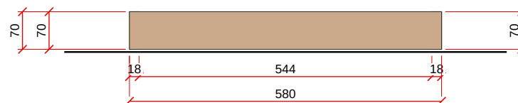
MÓVEL DIVERSO - ESC. 1:10
