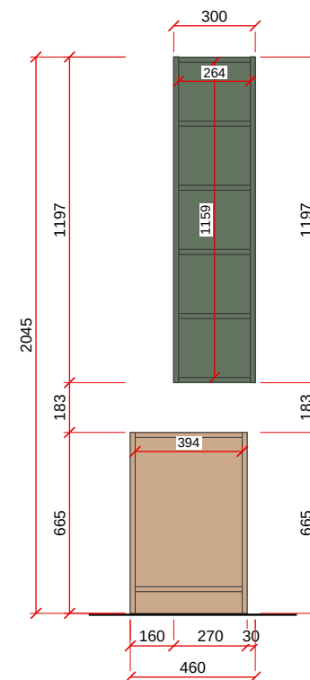
VISTA C - ESC. 1:25
