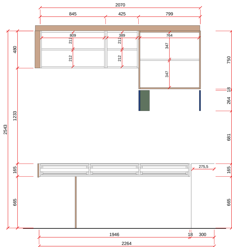
VISTA B - ESC. 1:25
